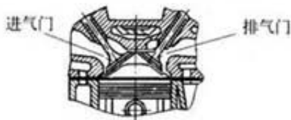
图7 活塞位于排气行程终了的上止点时进排气门叠开
