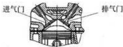
图6 活塞位于压缩行程终了的上止点时进排气门完全关闭
