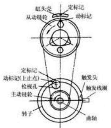
图5 飞轮上“T”标记与定标记对正时,从动链轮上的动标记与缸头上的定标记对正
