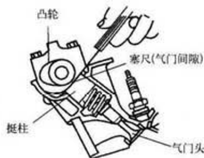
图4 直顶式配气机构的气门间隙
