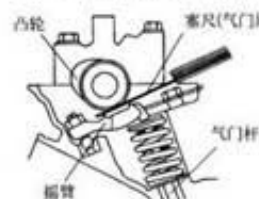
图3 下置摇臂式配气机构的气门间隙
